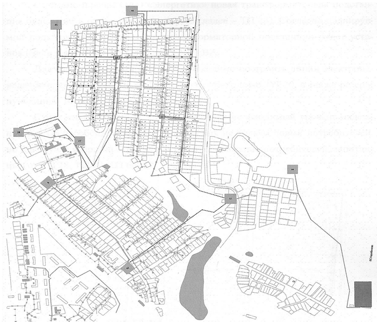
Рисунок - Схема электроснабжения ТП фидера Ф-1001.
